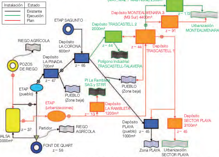
ESQUEMA ABASTECIMIENTO ALMENARA (Propuesta PGOU)
