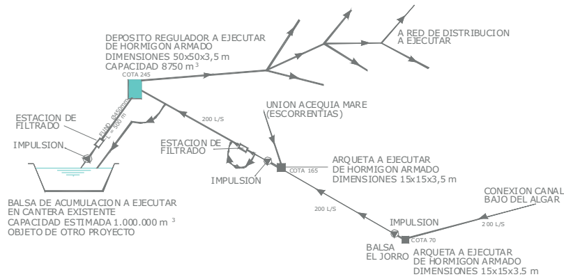
■ Esquema general de funcionamiento de la infraestructura hidráulica a ejecutar
