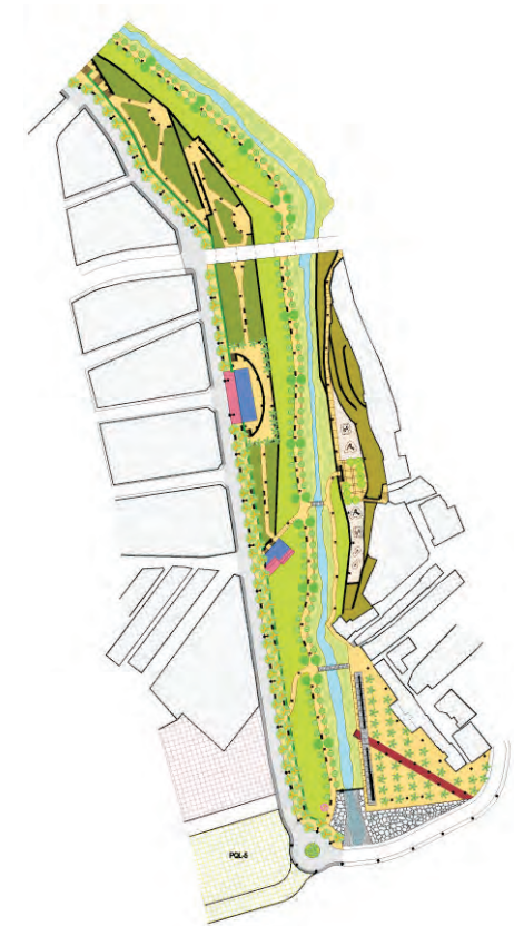
■ FASE IV. Planta general de la actuación
